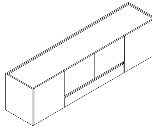
APARADOR 2 PORTAS E 2 GAVETAS 1800 x 480 x 400mm
